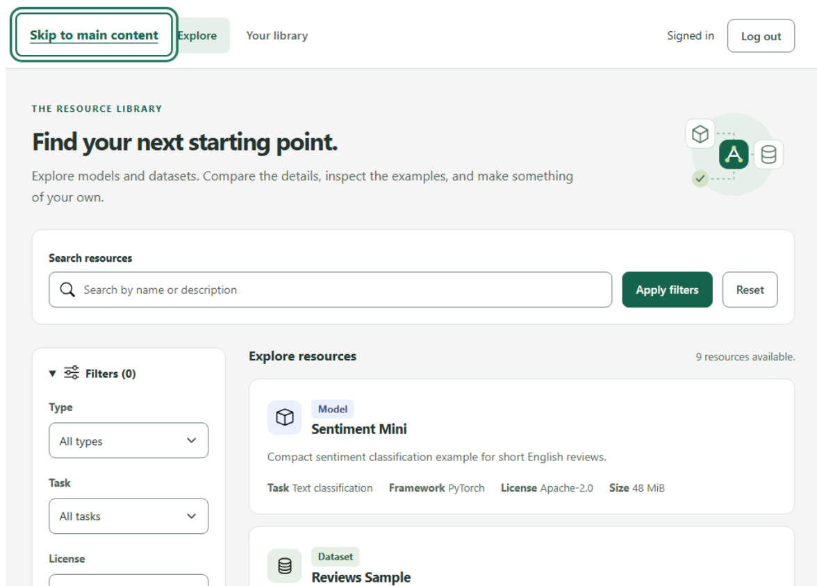
Рисунок 1. Видимый фокус на ссылке перехода к содержимому
